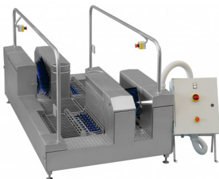
LAVE-BOTTES / SEMELLES INOX existe lave-bottes seul ou lave-semelles seul
